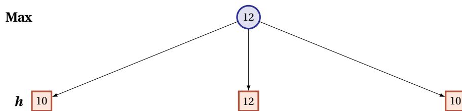
Exploration de l'arbre avec une profondeur de 1
